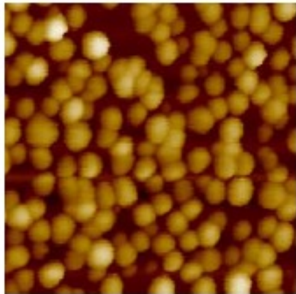
Au nanoparticle
